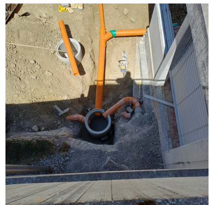
Pose des canalisations
